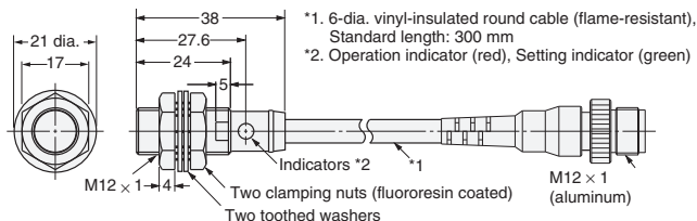
E2EQ-X10D1-M1(T)GJ
