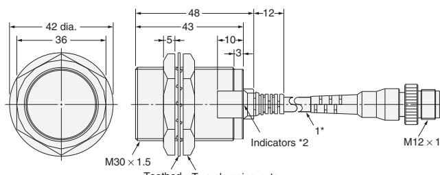
E2EQ-X15X1-M1(T)J
