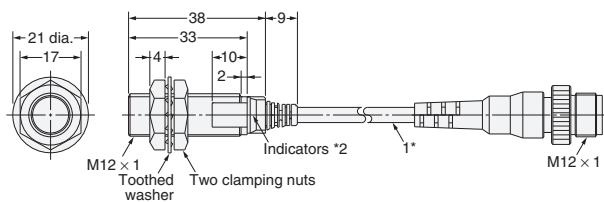
E2EQ-X4X1-M1(T)J
